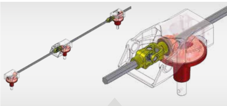
Meghajtás hatszög tengellyel és kardáncsuklós csatlakozásokkal
